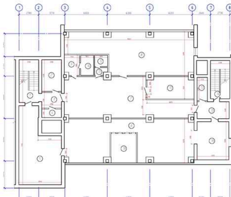
План подвала
