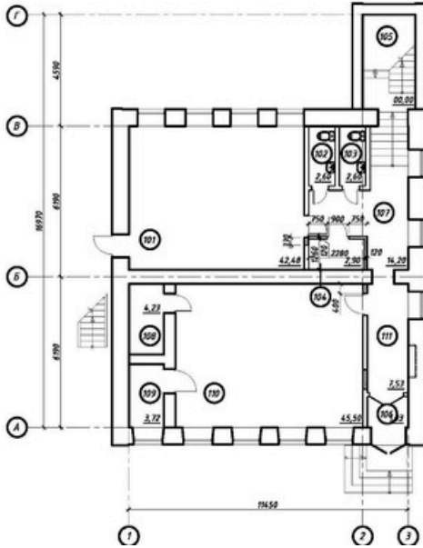
Проектируемый план 1-го этажа
