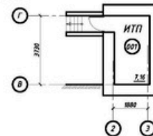
План подвала
