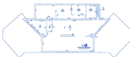
Планировка 2 этаж
