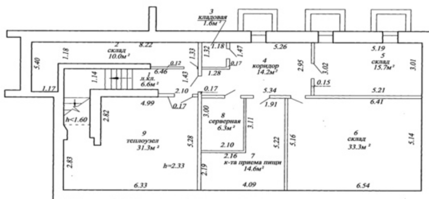
ПЛАН ПОДВАЛА
