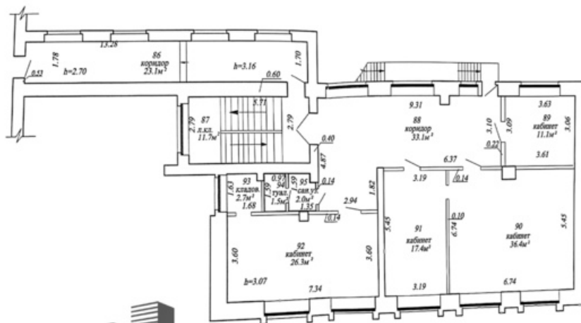
ПЛАН 3 ЭТАЖА
