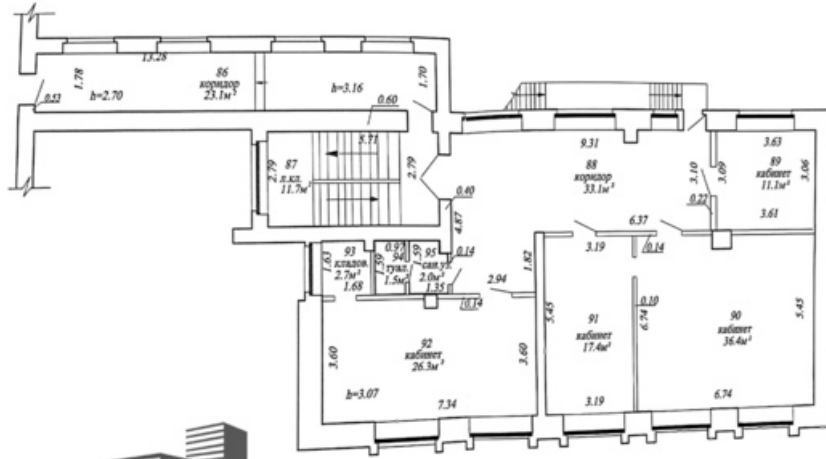
ПЛАН 3 ЭТАЖА
