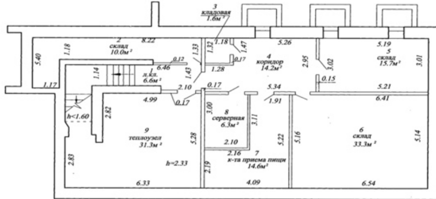
ПЛАН ПОДВАЛА
